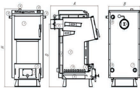
Рис.1 Magnum SF та його конструкція:
