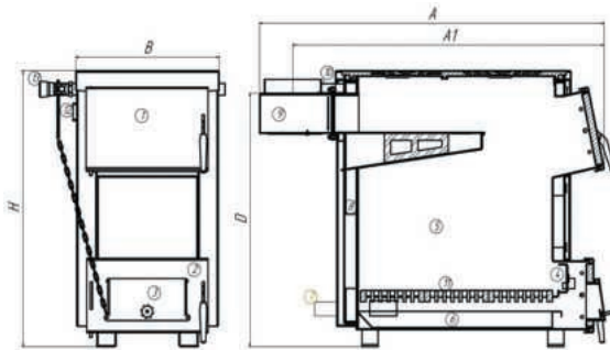
Рис.4 Magnum SF 20 та його конструкція:
