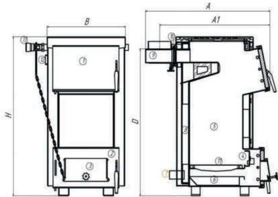
Рис.3 Magnum SSF та його конструкція:
