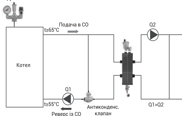
Рис.5 Схема з гідравлічним роздільником Група безпеки
